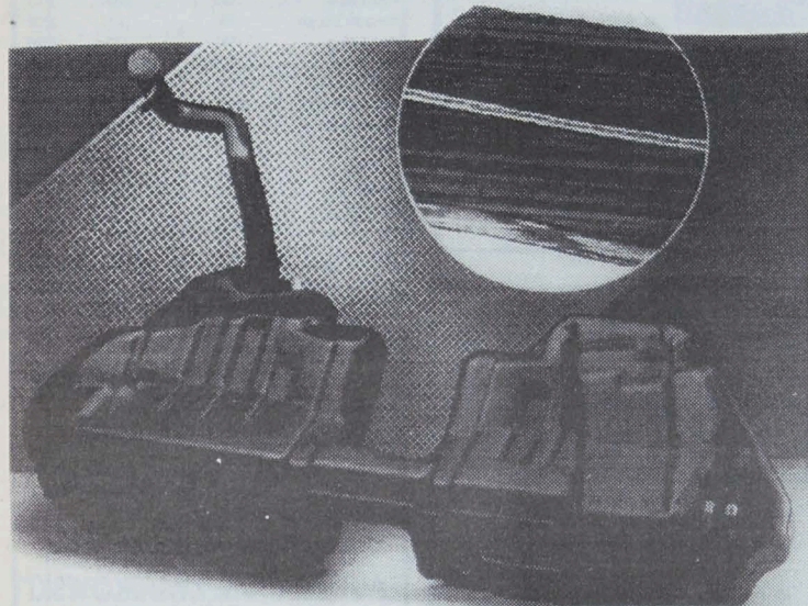
Tak wygląda sześciowarstwowy zbiornik paliwa do Mercedesa klasy C. Środkowa poprzeczka to miejsce na wał napędowy. Na fragmencie ścianki (w kółku) widać cienką warstwę uszczelniającą, tworzoną przez alkohol etylowy.
