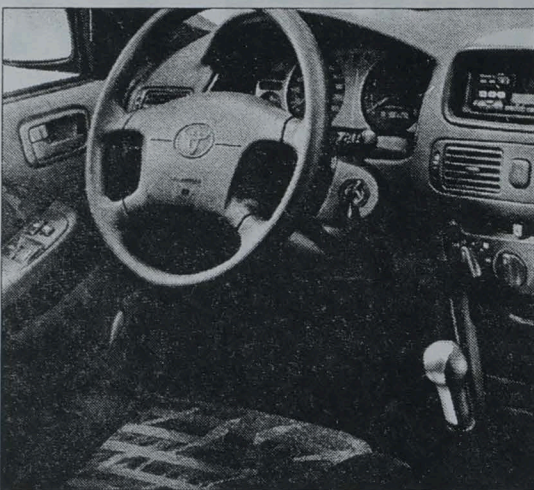
Miejsce pracy kierowcy w nowej Toyocie Corolli. Proszę zwrócić uwagę na panelowe rozmieszczenie elementów sterowania.
