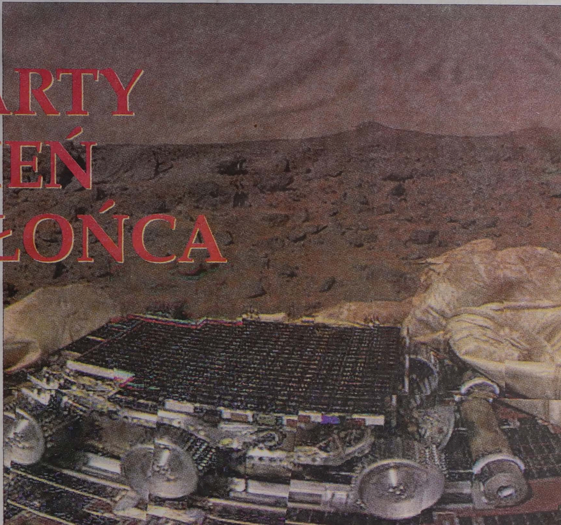
Krajobraz marsjański w barwach lososioowych. Niebo ma taki kolor z powodu unoszonych przez wiatry pyłów. Na pierwszym planie sonda Pathfinder. Na horyzoncie, w odległości 1,5 km od sondy, dwa wzgórza nazwane Twin Peaks.
