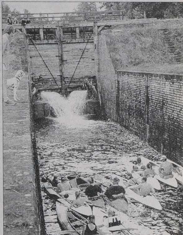
Dwukomorowa śluza w Paniewie
