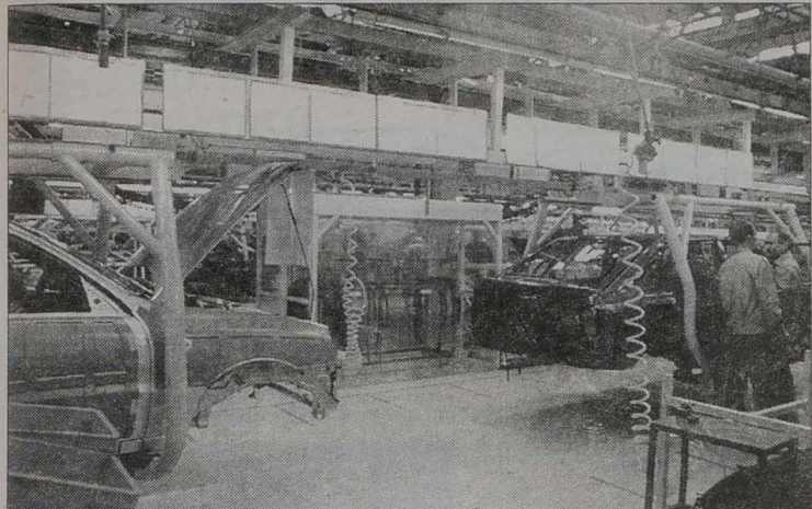
Podwieszane nadwozia Lanosów przemieszczają się wzdłuż linii montażowej wzbo- gacając się o kolejne podzespoły i instalacje
