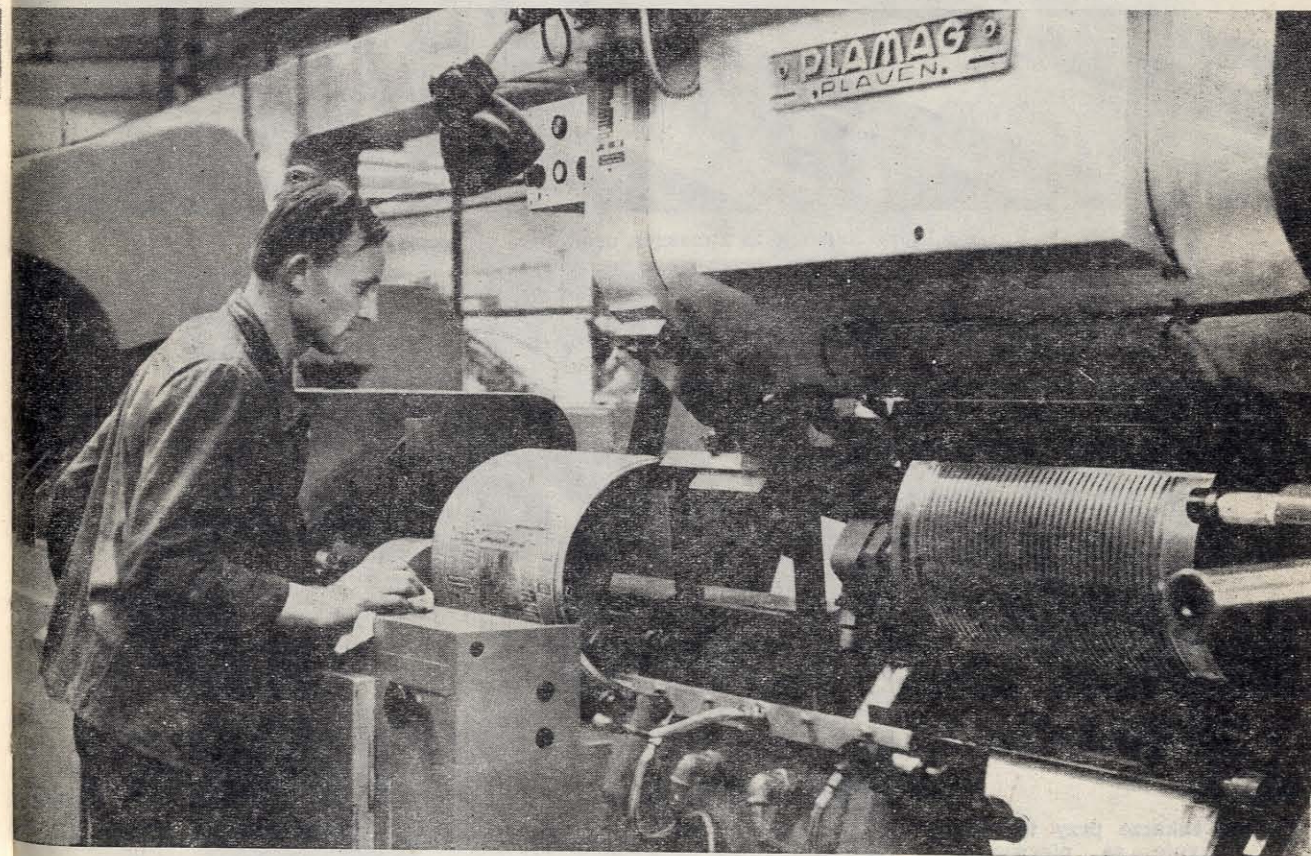
Maszyna odlewająca gazetowe „kolumny”, dopasowane do walców rotacyjnych.
