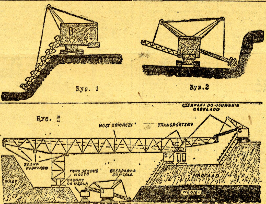
Na zdj. rys. 1 koparka kubelkowa, rys. 2 koparka kołowa, rys. 3 most zbiorczy w kopalni odkrywkowej.
