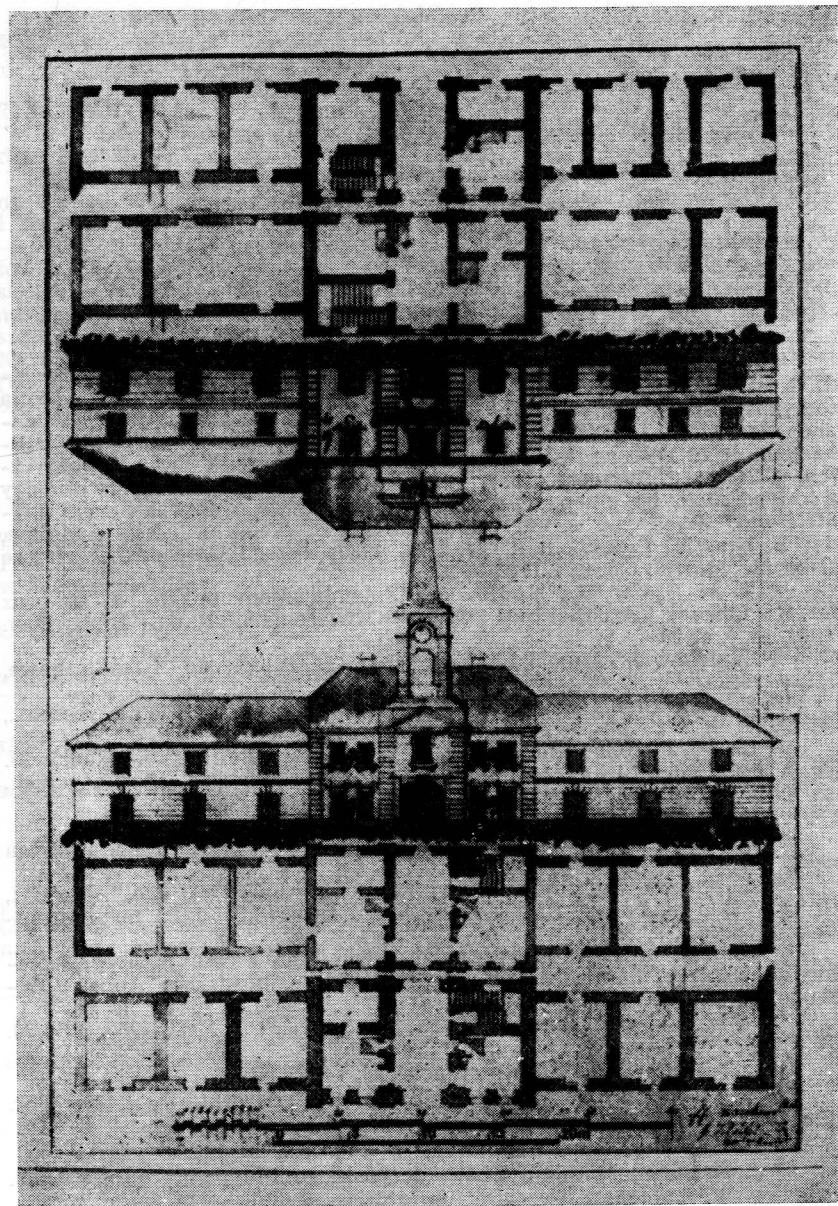
33. Ratusz w Siemiatyczach. Pomiar z ok. 1802 r. Oryginał w AGAD. U góry — rzut i elewacja skrzydła północnego, u dołu — skrzydła południowego.
