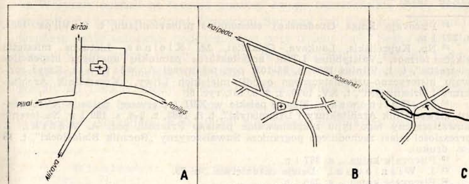
Ryc. 2. Przykłady rozplanowań miast litewskich z trójkątnymi rynkami według M. Kleinas
