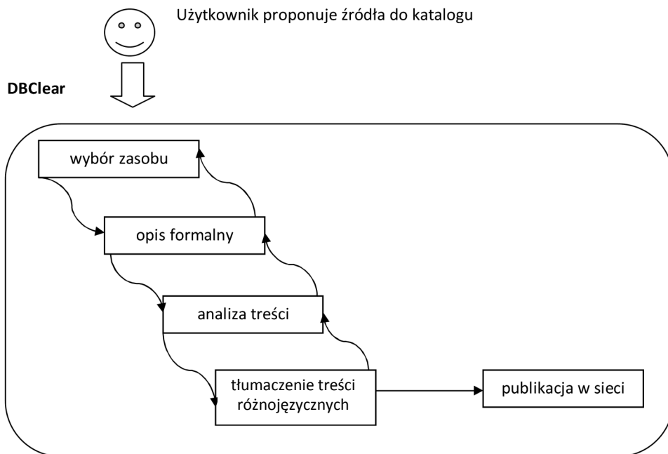
Ryc. 2. Przykładowy układ przepływu pracy w DBClear
