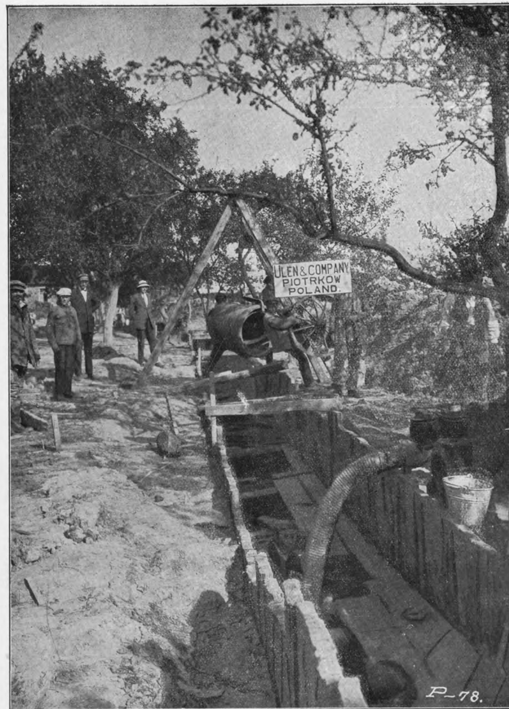
Fot. 5. Piotrków. Układanie rur kanałowych. (Str. 576).
