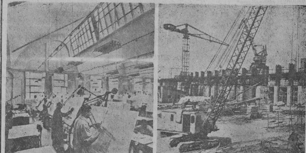
Gmach elektrowni, w którym znajdzie pomieszczenie 6 turbin wodnych o mocy 50 tys. kilowatów każda, będzie nie tylko fundamentem dla agregatów wodnych, lecz będzie również przyjmował na siebie ogromny napór wody. Większa część gmachu elektrowni znajdować się będzie pod wodą.
