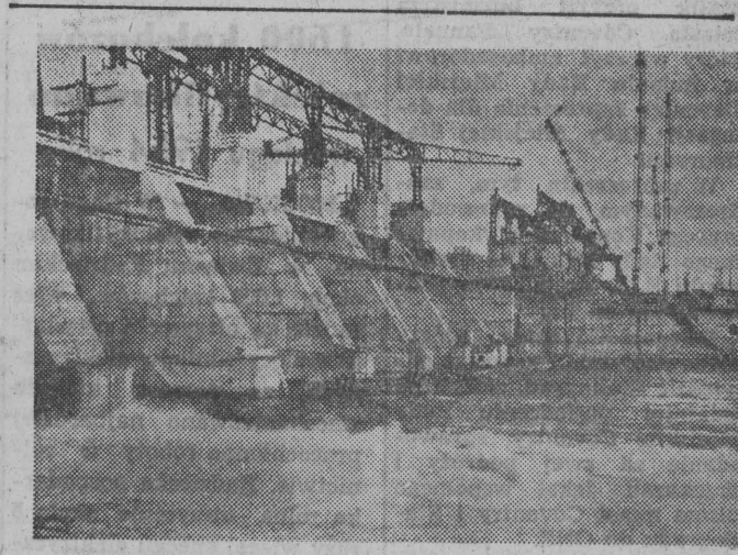
W Moldawskiej SRR trwa budowa Dubossarskiej Elektrowni Wodnej. Niedawno zakończono tu montaż pierwszego hydroagregatu. NA ZDJĘCIU: ogólny widok terenu budowy. Fot. — CAP
