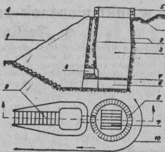
Piec Ślusarewa.
