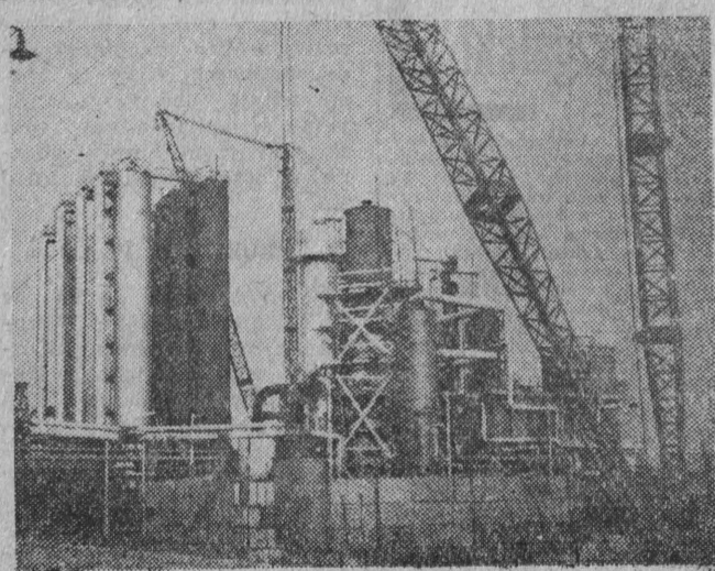
NA ZDJĘCIU: fragment działu benzolu w zakładach koksochemicznych hutnictwa im. Lenina. — fot. — CAF
