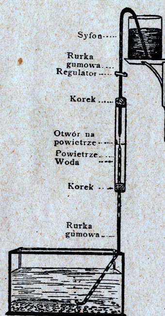
Przyrząd do przewietrzania wody.
