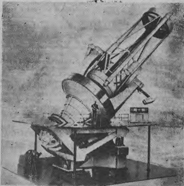
Wkrótce obserwatorium astrofizyczne na Krymie wyposażone zostanie w nowoczesny reflektor, którego konstruktorem jest laureat Nagrody Leninowskiej B. K. Joannisi-jan. Czynnny model nowego reflektora (zmniejszony 10 razy) wystawiony zostanie na wystawie w Brukseli.
