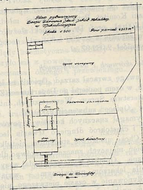
Plan sytuacyjny Domu zdrowia w Mikuliczynie.
