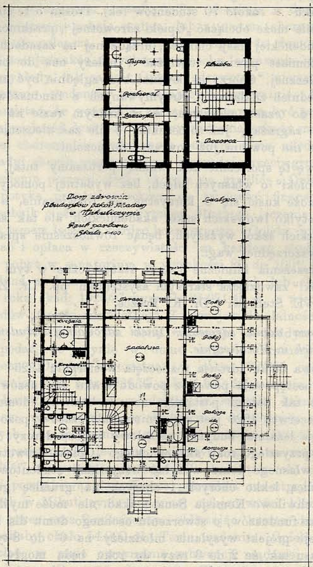
Plan Domu zdrowia w Mikuliczynie i budynku gospodarczego z krytem przejściem i leżalnią — rzut parteru.
