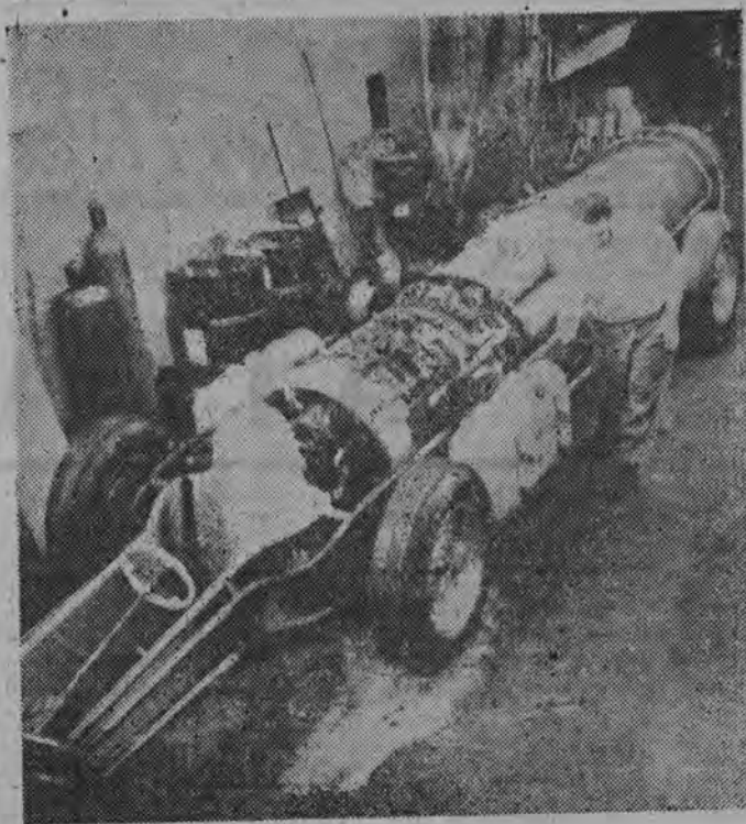
Kalifornijczyk Romeo Palamides skonstruował niezwykły polard, na którym chce pobić światowy rekord szybkości podczas małych cych się odbyć w sierpniu w Bonneville Salt Flat wyścigów. Samochód posiada silnik odrzutowy myśliwca F-86-D o mocy 16 tys. KM. Palamides i jego kierowca, były pilot Archie Leislerbrand, przypuszczają, że ich wóz wyścigowy może osiągnąć szybkość 720-1120 km. Do zatrzymywania samochodu na macie użyte zostały spadochrony.
