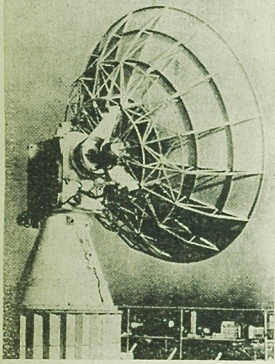
Francuskie urządzenie radarowe „BEARN” przeznaczane jest do śledzenia satelitów wyposażonych w radarowe urządzenia słowem lub ich pobawianych. W wypadku satelitów bez radarów nawigacja jest trudniejsza, 300 km od celu poruszającego się z szybkością 18 000 m/s. Polaryzacja w radar anten 18 000 m/s odległości 400 km.
