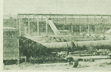
NA ZDJĘCIU: piece przetapiające wydziału tlenku cynku.
