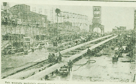
Tak wygląda pochylina stoczni przed położeniem na niej stępki pod przyszły statek.
