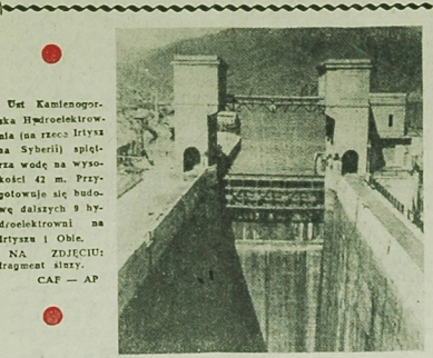
Ust. Kamienoproska (na rzecze Irtysz na Syberii) przystąpiła w 1967 r. do budowy dużego elektrowni na Irtyżu i Obie.
