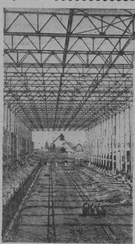
NA ZDJĘCIU: budowa oddziału żelazowego z elementów prefabrykowanych. CAF
