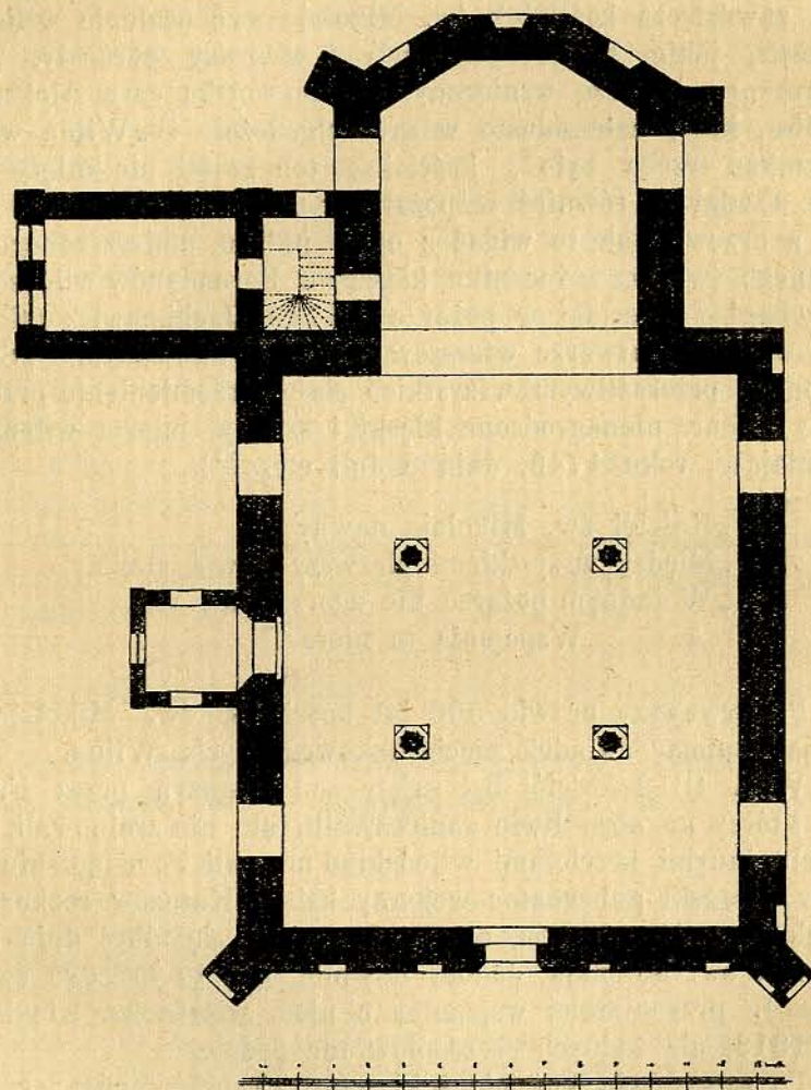
Plan Kościoła Św. Mikołaja; wykonał Stanisław Dąbrowski.
