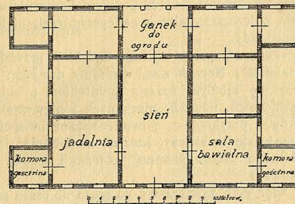
Rozkład starożytnego dworu w Kowalewsczyźnie na Podlasiu. (Z „Budownictwa drzewnego“ Z. Glogera).
