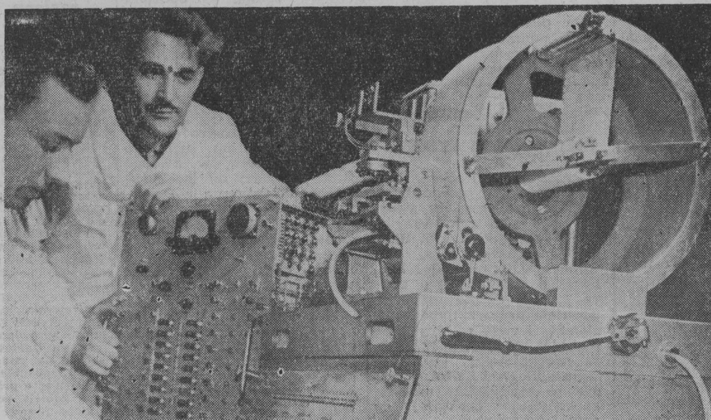
W moskiewskiej fabryce „Nietiepribor” produkującej sprzęt do poszukiwań złóż ropy naftowej i gazu ziemnego, zakończono montaż nowej aparatury sejsmicznej (na zdjęciu), która wkrótce zostanie zastosowana do badań roponośnych okęgów ZSRR.
