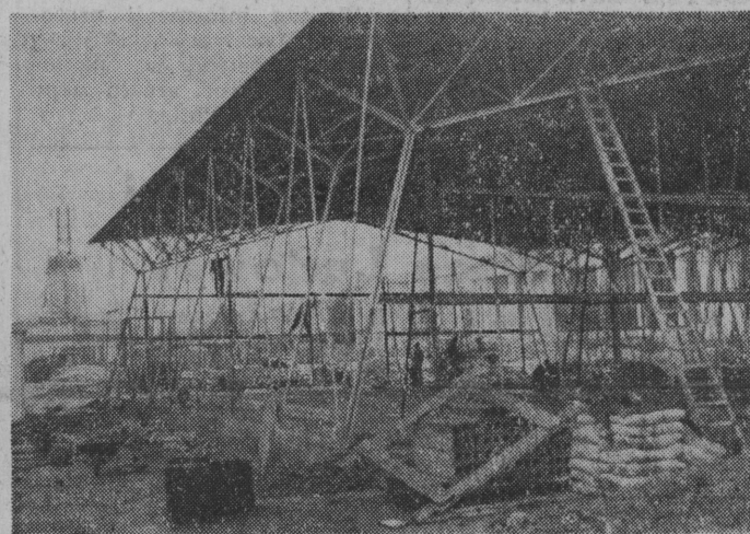
Na terenach targowych w Poznaniu trwają intensywne prace przygotowawcze do XXXIII MTP. M. in. w centrum terenów wystawowych buduje się nowoczesne efektywne pawilony ze szkła i aluminium. NA ZDJĘCIU: fragment budowy pawilonu jugosłowiańskiego. CAF — fot. Staszyszyn
