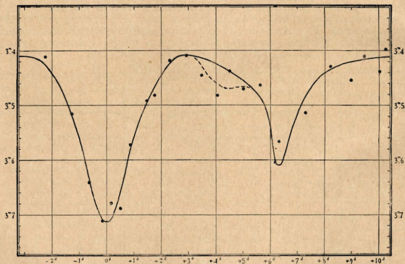
Rys. 2. Krzywa zmian blasku \beta Lyræ.
