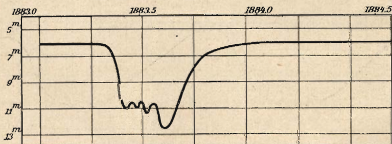
Rys. 8. Krzywa zmian blasku R Coronae Borealis, przykład gwiazdy częściowo regularnej. Na osi poziomej oznaczono lata.
