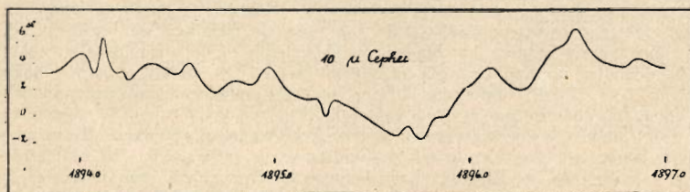
Rys. 10. Krzywa zmian blasku \mu C e p h e i, według obserwacji z lat 1894 — 1897. Jasności wyrażone są w stopniach. Blask gwiazdy zmienia się w gminach 4 m .0 — 4 m .8.
