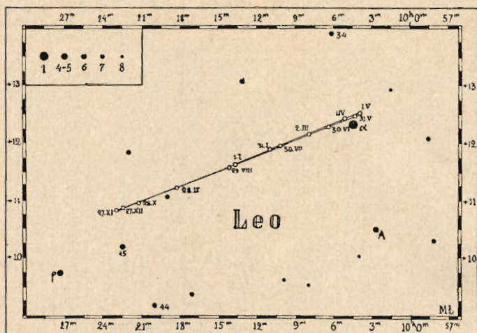
Pozorna droga Neptuna wśród gwiazd w r. 1929.
