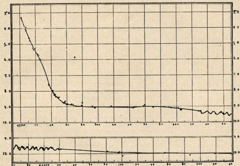
Rys. 9. Krzywa Nowej C y g n i III (r. 1920) według obserwacji dokonanych w Polsce. Liczby na osi poziomej oznaczają daty, wyrażone w dniach t. zw. nowej ery astronomicznej. 43700 = 1920 r. VIII 24 d ; 44000 = 1922 r. VII 13 d ).
