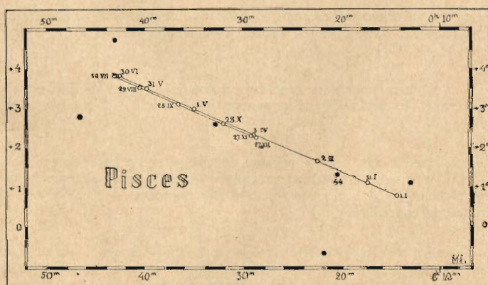
Pozorna droga Urana wśród gwiazd w r. 1929.
