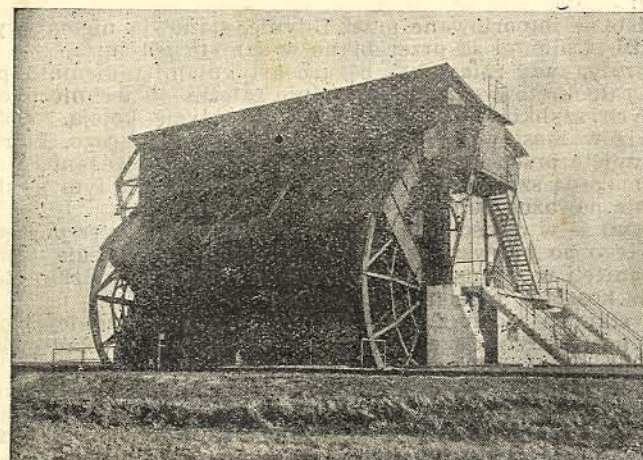
Port w Gdyni. Transporter węglowy. Wywrotnica wagonów.
