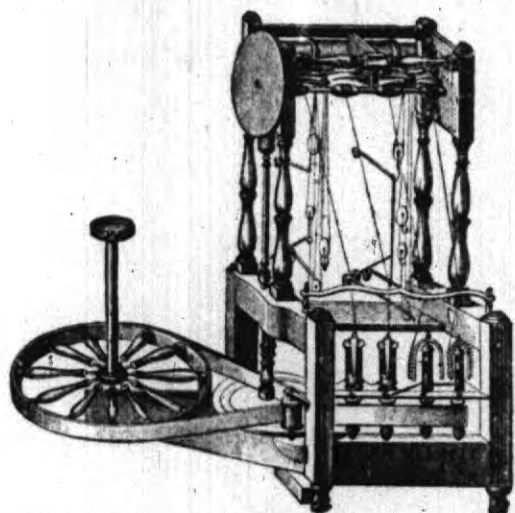
Warsztat tkacki Arkwright'a, poruszany siłą wody (1769).
