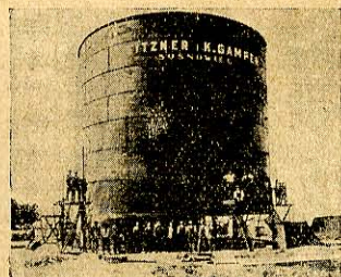
Zbiornik na wodę 14 m. średnicy i 13 m. wysokości dla Magistr. m. Radomia
