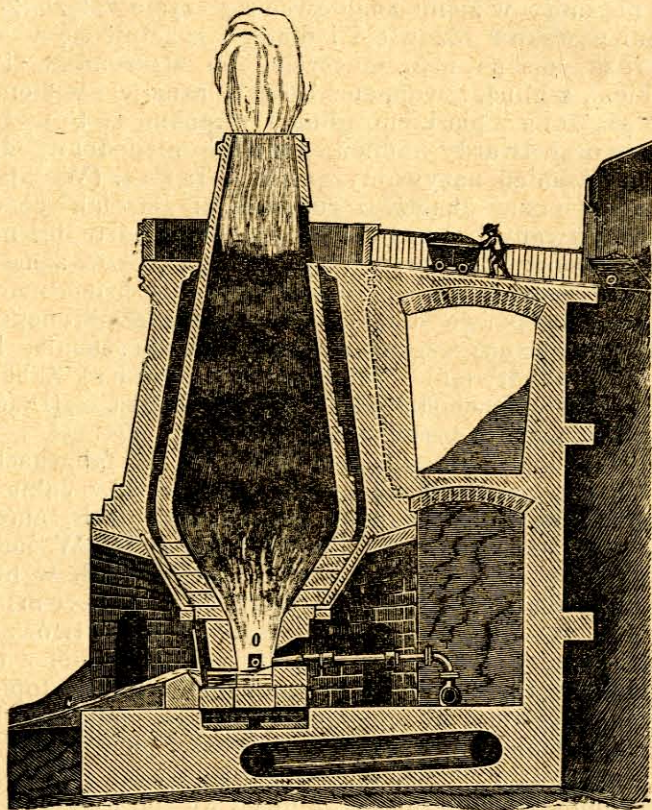
Rys. 41. Przecięcie wielkiego pieca w hucie żelaznej.
