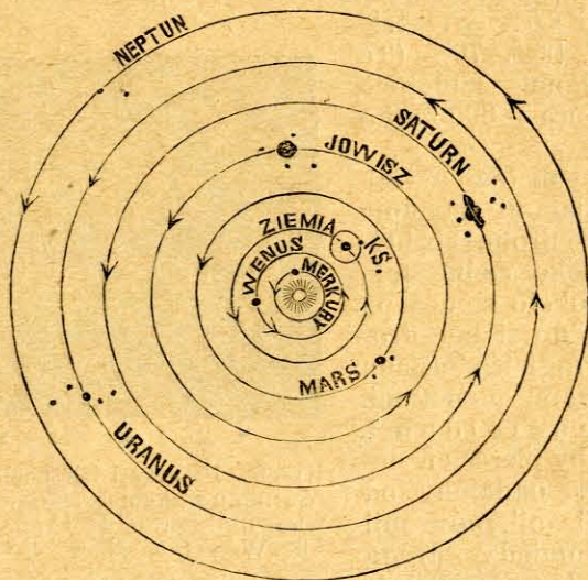
Rys. 70. Porządek obiegu planet około słońca.
