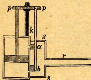
Rys. 58. Drażek otwierający zamykający kłapy w cylindrze.
