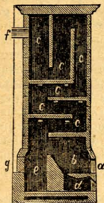
Rys. 64. Przecięcie pieca kaflowego: a —drzwiczki, b —palenisko, d —popielnik, oddzielony od paleniska rusztem, e —miejsce, w którym zbierają się sadze, popiół, porwane przez ciąg, wygarniają się lufem, g , cccc —kanały, f —ujście do komina, zamknięte szybem w piecach zwyczajnych, bez zamknięcia — w hermetycznych.
