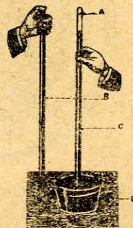
Rys. 62. Przyrząd do mierzenia ciśnienia powietrza: B rurka szklana barometryczna z rtęcią, C ta sama rurka z rtęcią, zanurzona w wannie D z rtęcią, A. próżnia po rtęci opadłej.
