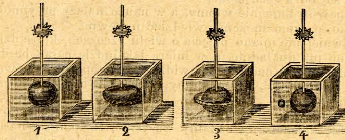
Rys. 75. Doświadczenie z kroplą oliwy, obracaną wokół jej osi.
