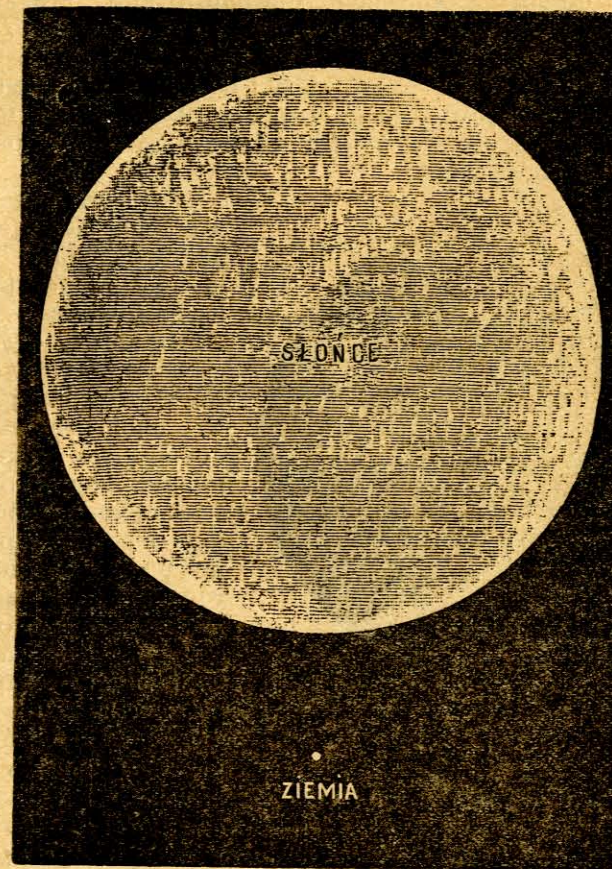
Rys. 71. Stosunkowa wielkość słońca i ziemi.
