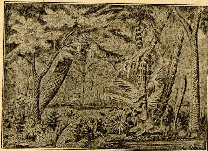
Rys. 30. Las pierwotny (widłaki, paprocie i skrzypy).
