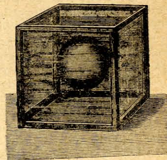
Rys. 49. Kropla oliwy przyjmuje kształt kulisty.
