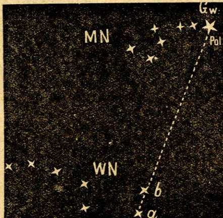
Rys. 74. Gwiazdozbiory Wielkiej Niedźwiedzicy (u dołu) i Małej Niedźwiedzicy (u góry). Gwiazda większa u góry jest Gwiazdą Polarną.
