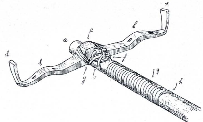
4. Jochverband am homerischen Wagen (Wiederherstellung).
