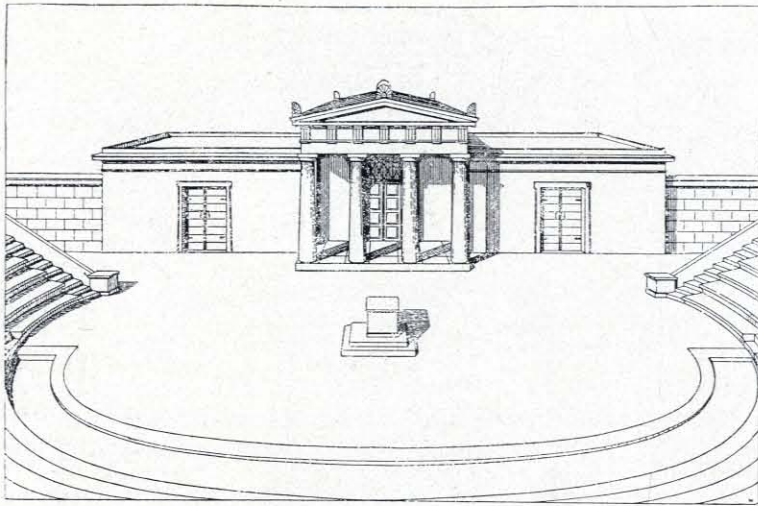
1. Dreiteiliges Spielhaus (Skene) mit Vorhalle, V. Jahrh.
