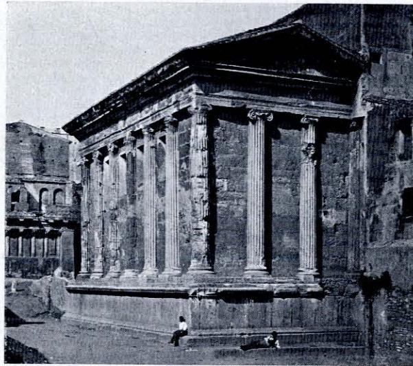
2. Tempel der Fortuna virilis zu Rom.
