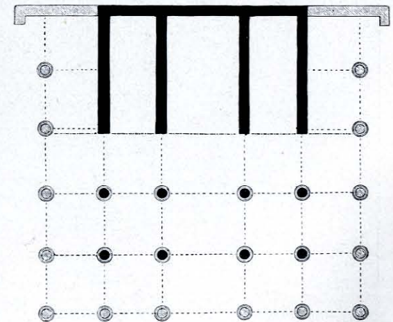
5. Jupitertempel (Grundriß).
