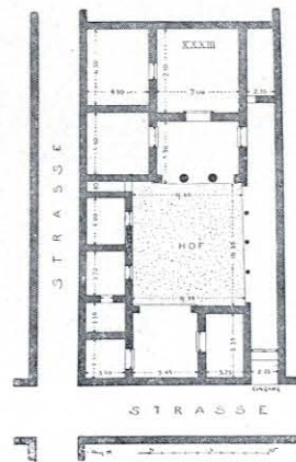
3. Haus in Priene — Grundriß und 4. Wiederherstellung.
