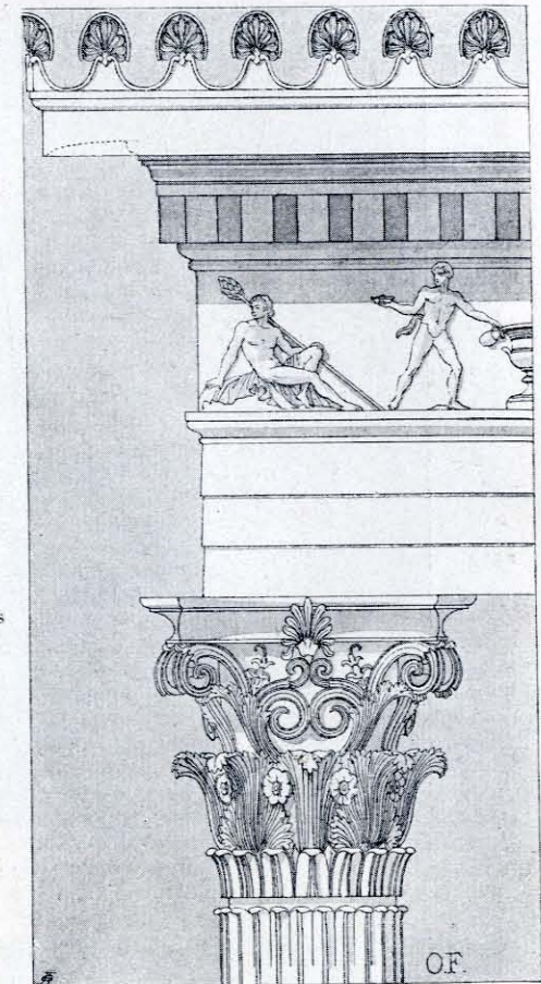
3. Korinthische Säule.
