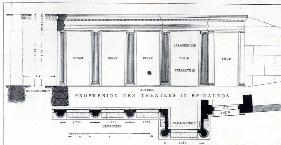
3. Vorbau des Spielhauses (Proskenion) im Theater zu Epidauros (Wiederherstellung).
