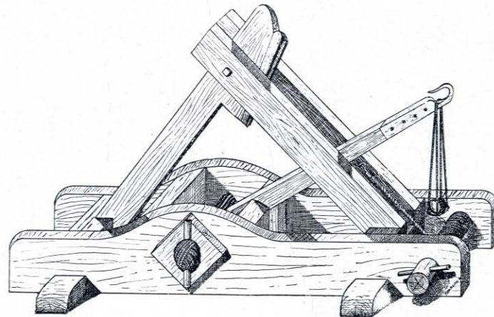
3. Schleuder für schwere Steine — funda librilis.
