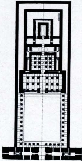
1. Grundriß.
