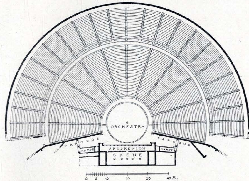
2. Grundriß des Theaters in Epidauros, ergänzt.
