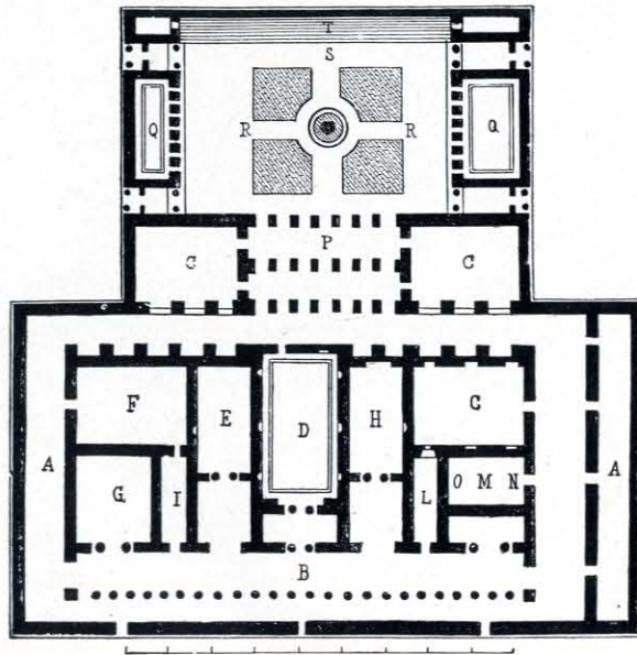
2. Gymnasium zu Hierapolis.
