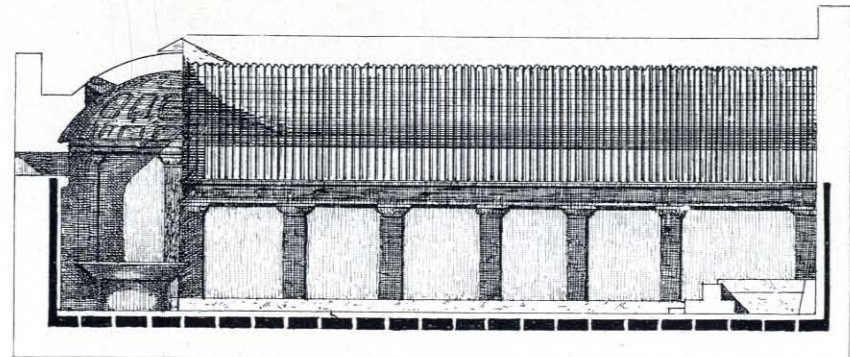
3. Caldarium der Forumthermen (Durchschnitt).
