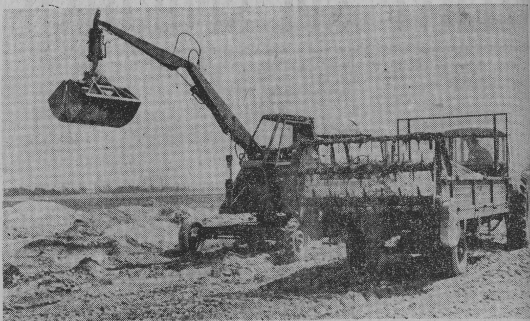
W Kindzienku k/Błonia prowadzi się badania nowych maszyn rolniczych. NA ZDJĘCIU: roztrzaskacz obornika, przystosowany do rozsiawu wapna nawozowego. Zmechanizowanie wapnowania gleb jest jednym z ważniejszych problemów również na Białostocczyźnie.
