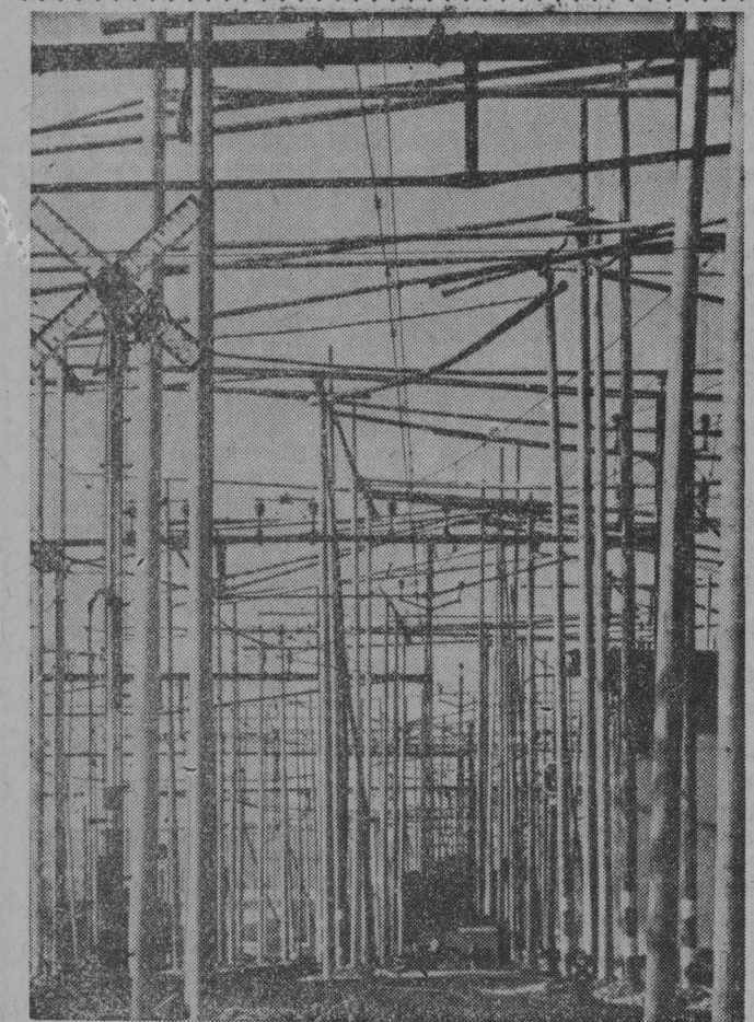
Ten las masztów znajduje się na szwajcarskiej stacji kolejowej Muttentz, ważnym węźle kolejowym i ma za zadanie zapobieganie katastrofom na tej ruchliwej stacji w wypadku zerwania się sieci wysokiego napięcia. CAF
