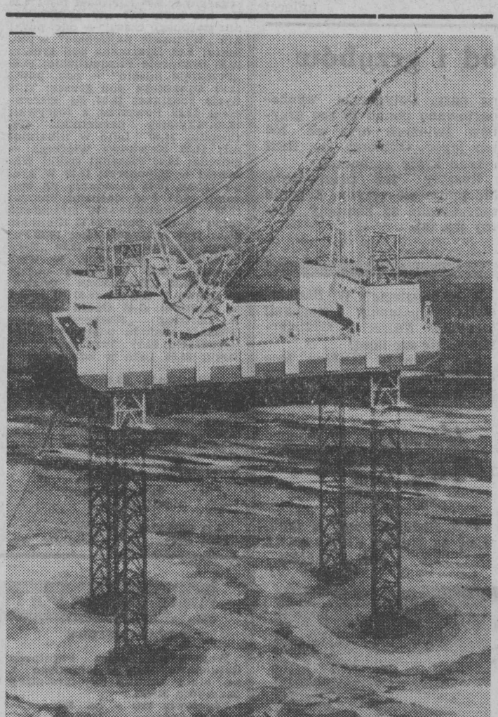
Największa na świecie platforma przeznaczona do naprawy pływających wież wiertniczych, zbudowana zostanie w zakładach Nagoya w Japonii na zamówienie koncernu naftowego Aramco Overseas G. i zainstalowana w Zatoce Arabskiej wiosną 1977 r. Długość platformy wynosi 80 m, szerokość — 36 m, wysokość — 7 m, a jej ciężar szalony jest podnieść 500 ton.
