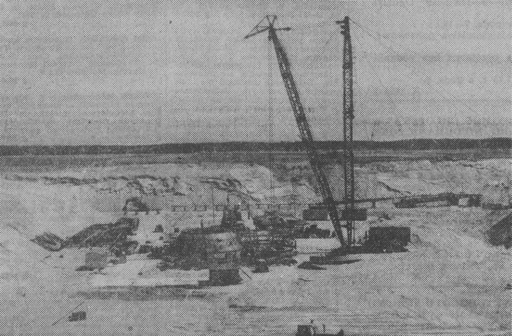
Montaż gigantycznej koparki o wydajności 1 tys. ton wrobku na godzinę pracy. Aby ustawić koparkę w odkrywcę, wydobyto stąd prawie półtora miliona m sześciu ziemi.
