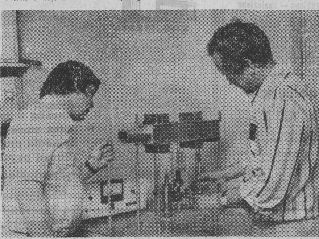
NA ZDJĘCIU: (od lewej) Henryk Zak i dr inż. Andrzej Chachulski — kierownik Pracowni Atomowych Wzorców Czystości — i T — przy zminiaturyzowanym laboratoryjnym modelu wzorca. CAF — Rosiak
