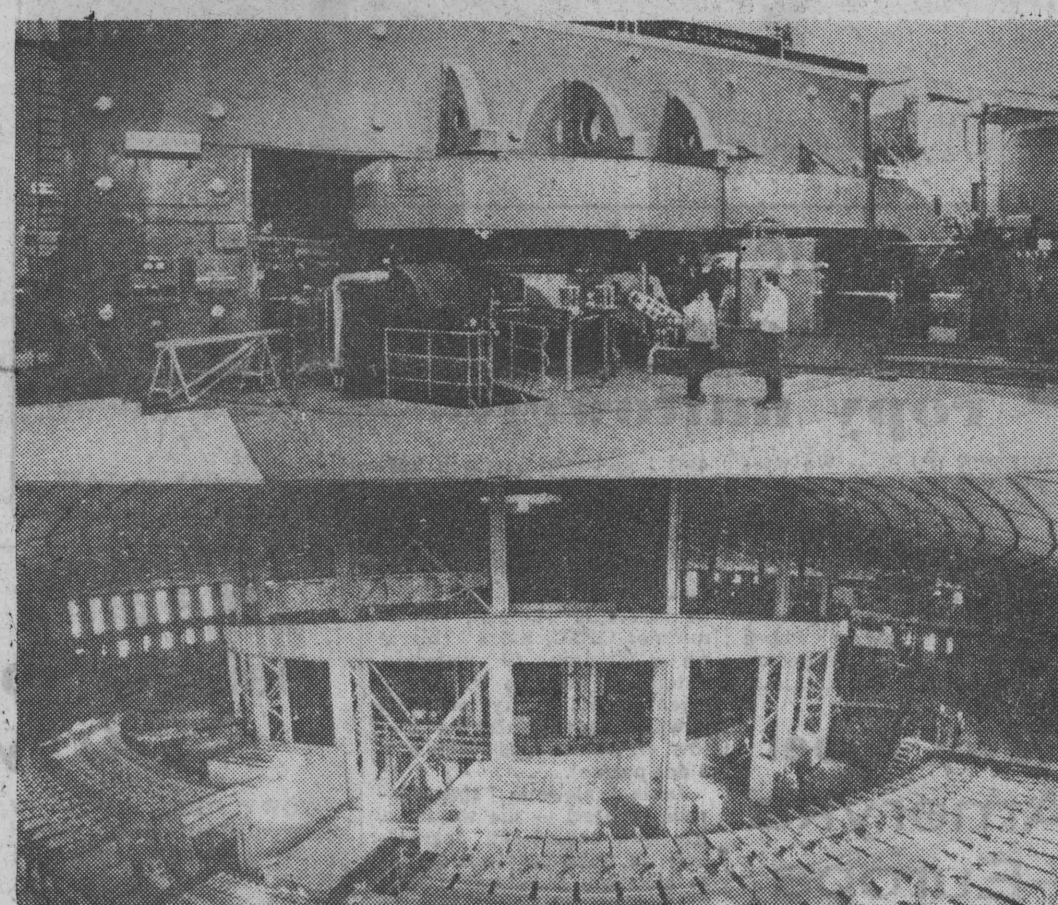
NA ZDJĘCIU: góra. Pierwszy eksperyment Instytutu Badań Jądrowych w Dubnie pod Moskwą uruchomiony został w 1959 roku. Dół: synchrotron Instytutu. Jego ogromny magnes o średnicy 50 metrów waży 35 ton. CAF — TASS
