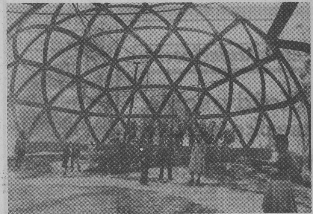
Gigantyczna ptaszarnia o długości 21 m, szerokości 15 m i wysokości 10 m zbudowana została w parku St. Vrain w Paryżu, według planów architekta H.W. Mullera. Ten uniwersalny pod względem wielkości obiekt — to plastikowa kopuła wsparta na stalowej konstrukcji, pierwsza tego typu ptaszarnia z naturalnym oświetleniem. CAF—AFP
