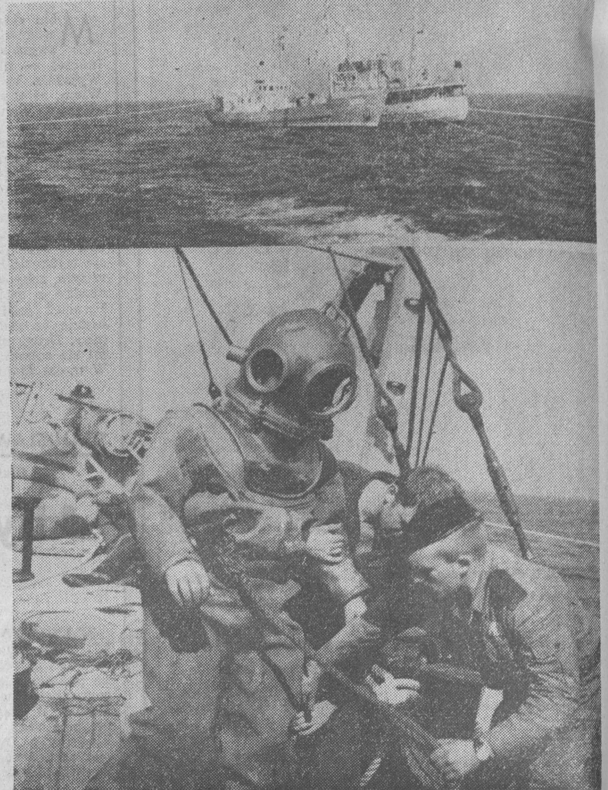
NA ZDJĘCIU: (u góry) statek badawczy CMM „Wodnik” i okręt ratowniczy Marynarki Wojennej „R-21” zakotwiczone nad wrakiem „miedziowca”; (u dołu) nurk bosman Franciszek Marek przygotowujący się do kolejnego zejścia pod wodę do wydobywania następnej partii ładunku „miedziowca”.
