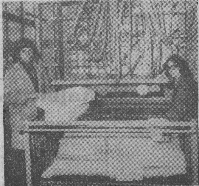
Mikołaj Ostrowski i Emilia Szczepanowicz obsługują automat wytwarzający opakowania ze styropianu.
