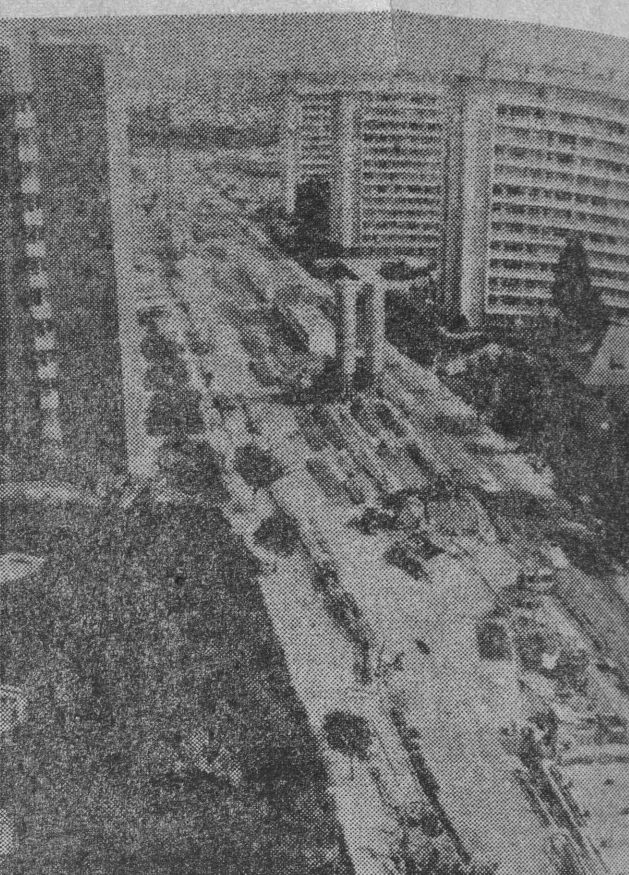
BELGIA. Budowa nowego odcinka brukselskiego metra w dzielnicy Woluwe St. Lambert. CAF — Belgia
