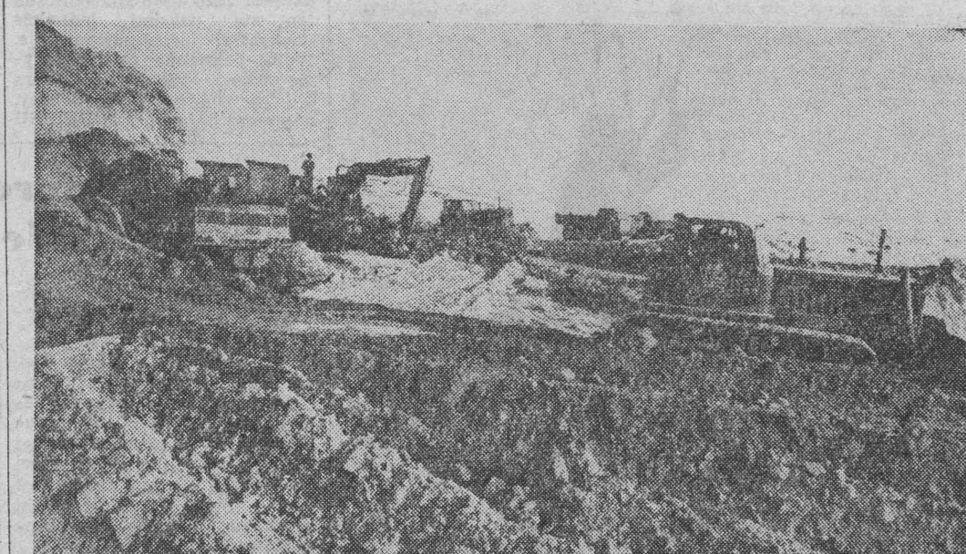
NA ZDJĘCIU: prace niwelacyjne na linii hrubieszowskiej.
