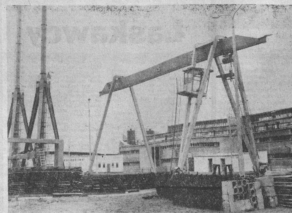
Plac składowy Fabryki Domów w Oleku przygotowany jest do przyjęcia pierwszej partii prefabrykatów. W ich przemieszczaniu i załadunku na środki transportowe, pomagają będzie suwnica bramowa. W głębi główna hala produkcyjna zakładów. Fot. Z. Zaremba
