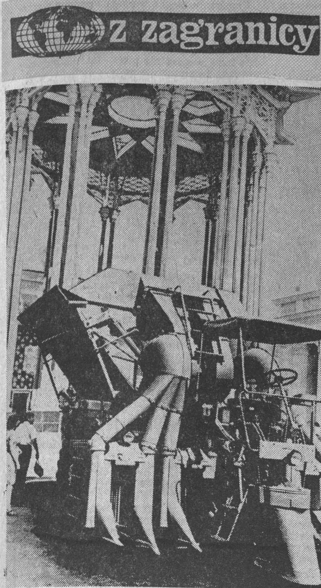
Na wystawie osiągnięć gospodarczych ZSRR w Moskwie zaprezentowano nowy model kombajnu do zbioru bawełny uprawy z krzaków, produkcyjnej radzieckiej fabryki Taszelmaz z Taszkentu. Nowa maszyna — KNE — 3,6 zbiera bawełnę zbierakiem szerokości 3,6 m rosnącą w rzędach odległych od siebie na 90 cm. CAF—TASS
