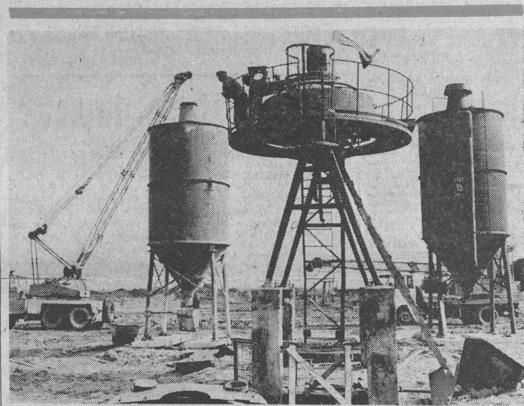
NA ZDJĘCIU: budowlani instalują urządzenia do wytwarzania betonu.
