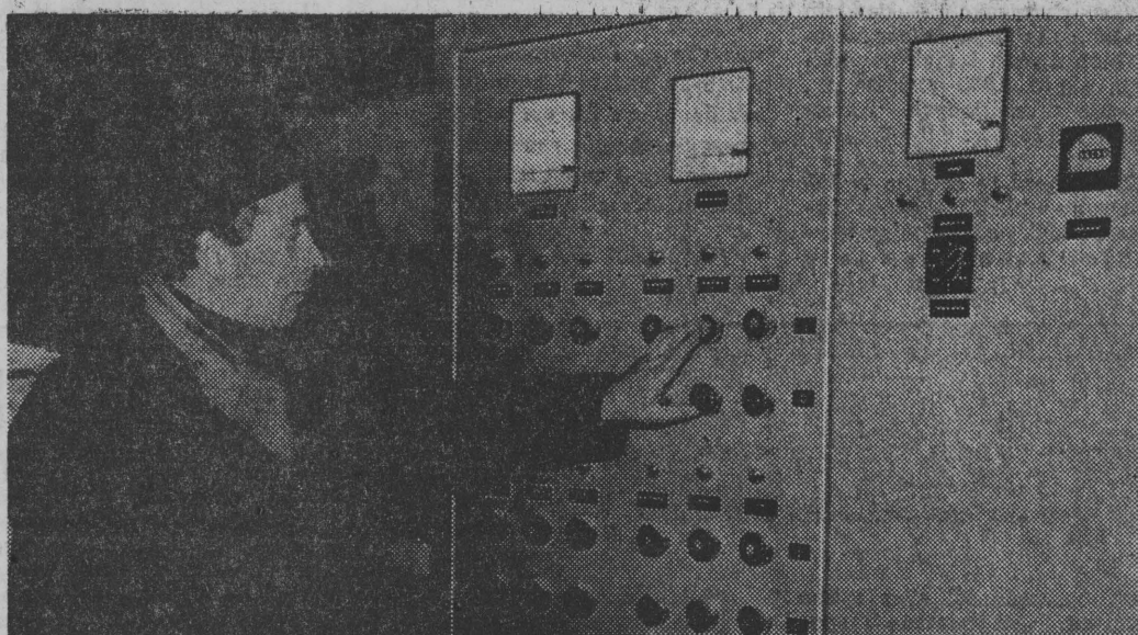
Pulpit sterowniczy linii technologicznej do produkcji pasz pełnoporcjowych na bazie słomy obsługujący Józef Michalczyk.
