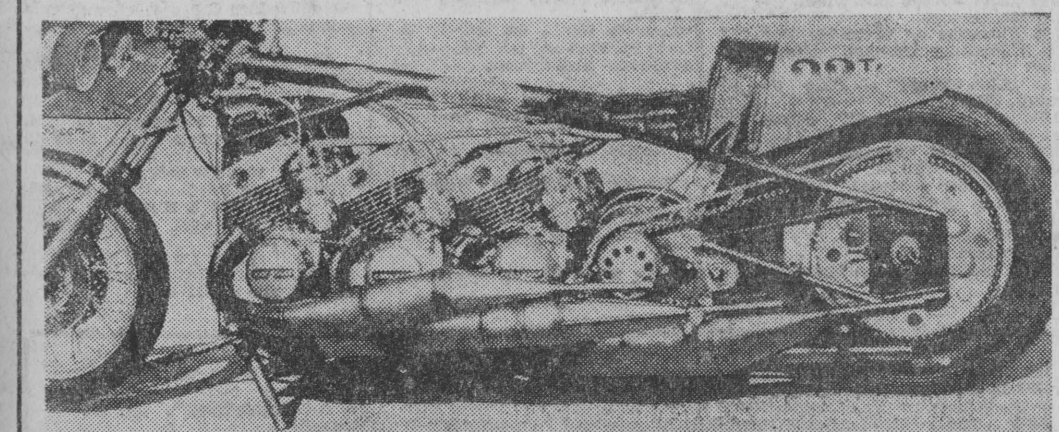
Motocykl monstral, Denso-Kawasaki, najszybszy z motorów napędzanych normalnym paliwem. Na wyścigu osiągał szybkość 800 km/h.
