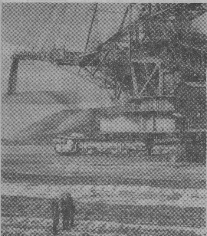
Z kopalni węgla brunatnego w Bełchatowie wydobyto już ponad 16 mln metrów sześciennych nadkładu, przykrywającego pokłady węgla. Ziemię zbiera od czerwca ub. roku ołbrzymia koparka o ciężarze ponad 7 tys. ton. CAF—Zbraniecki—teletfoto
