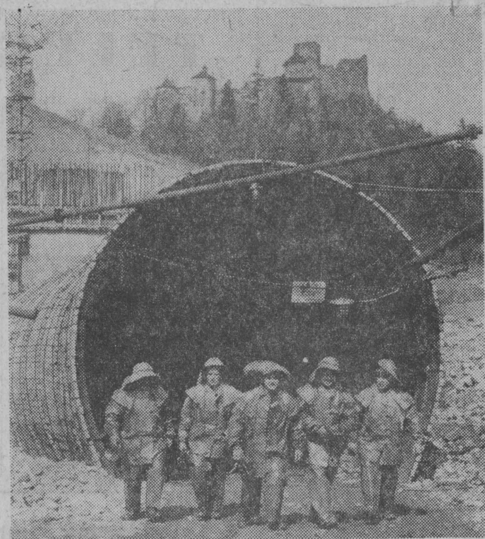
NA ZDJĘCIU: budowa zapory na Dunajcu. CAF — Momot
