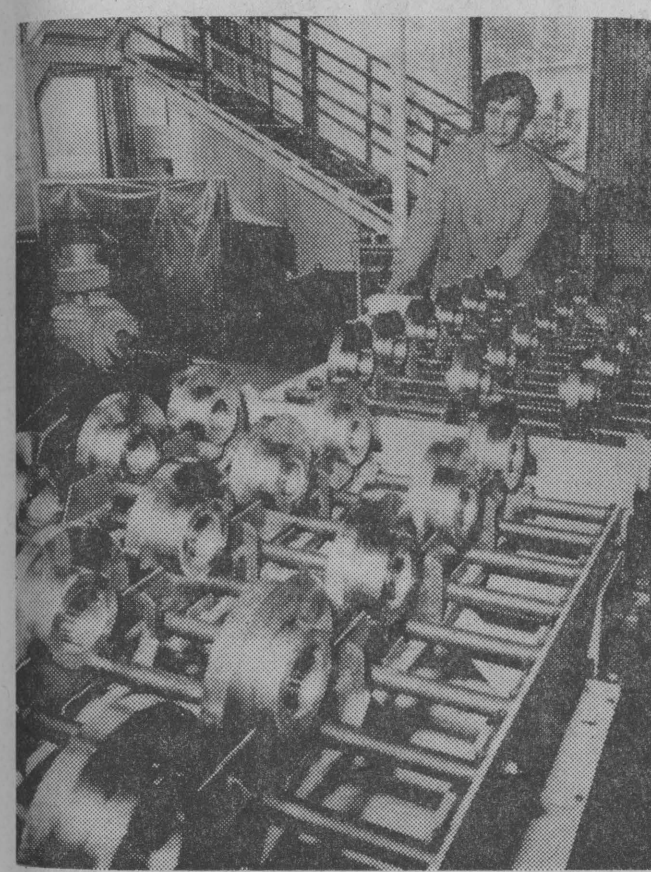
BULGARIA. Numerycznie sterowane urządzenie transportu wewnątrzzakładowego opracowane w sofiskim instytucie budowy obrabiarek. Urządzenie to transportuje z magazynu na halę produkcyjną detale maszyny znaczące u- sprawniających pracę.
