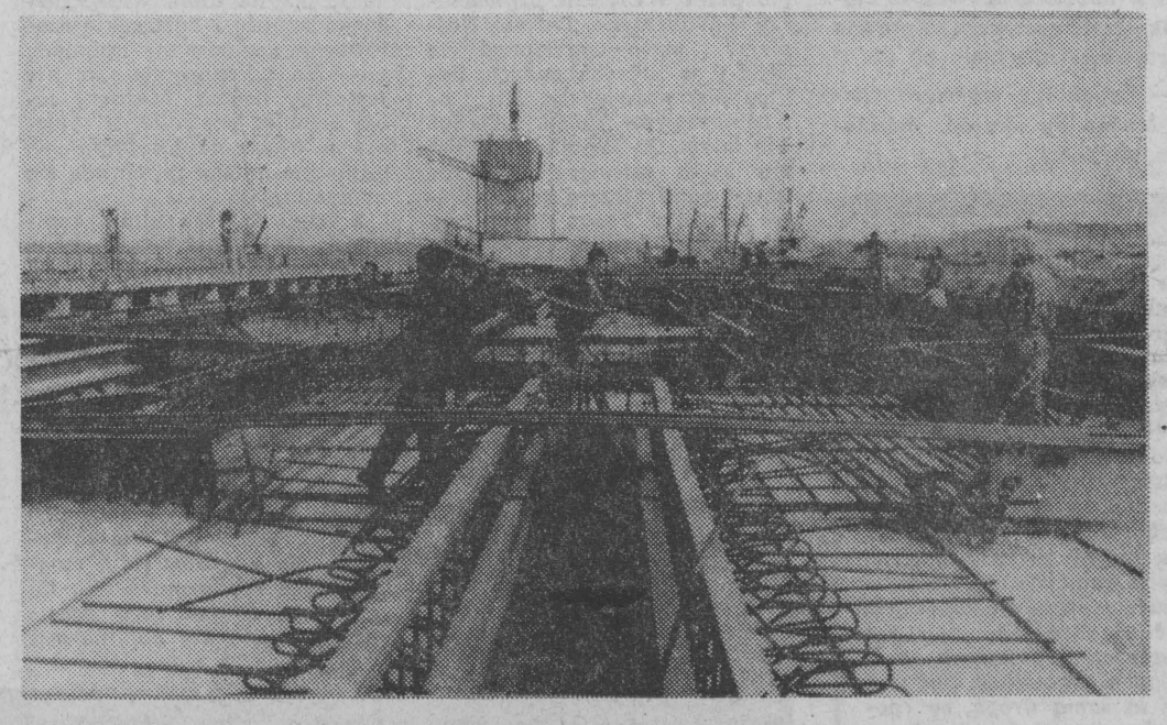
Betonowanie fundamentów pod pierwszy i drugi kotłowni. Elektrowni w Rogowcu.
